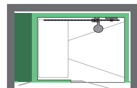
Nischeneinbau mit Sichtschutzwand und Technikraum
