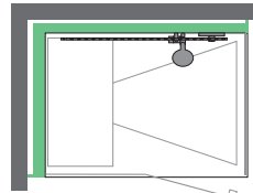
Eckvariante mit Glasfront, Technik extern
