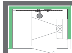
Installation en angle avec façade vitrée
