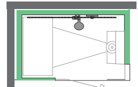
Installation en angle avec paroi pare-vue
